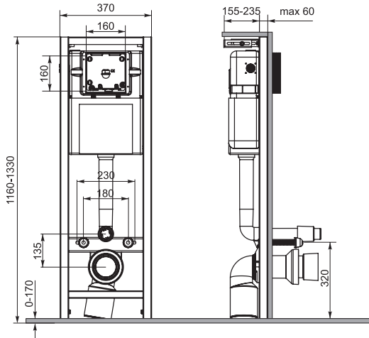
Креслення Nest UNI QT0233M370
