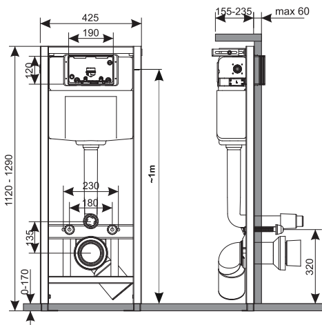
Креслення Nest QT0133M425
